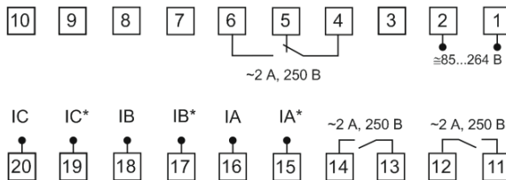
Рис. 4 – Клеммы подключения
