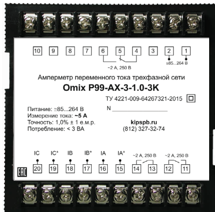
Рис. 7 – Задняя панель прибора
